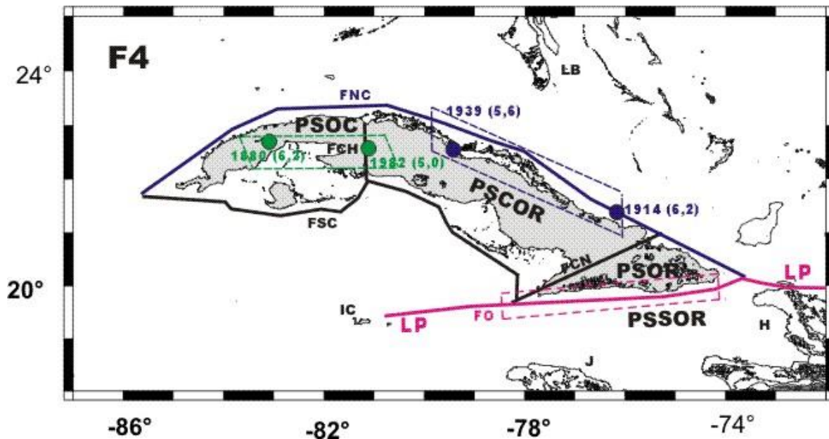
Figura 4.- Provincias Sismotectónicas y áreas con eventos sísmicos más fuertes. 1) Provincia Sismotectónica (PSOC= Occidental, PSOR= Centro Oriental, PSOR= Oriental, PSOR= Suroriental); 2) Límites de las Provincias (fallas activas: 2.1) líneas negras con siglas: FCH= Cochinos, FCN= Cauto-Nipe, FSC= Surcubana; 2.2) línea morada con sigla FNC= Nortecubana; 2.3) línea roja con sigla FO= Oriente; 3) Áreas con eventos sísmicos más fuertes por Provincia Sismotectónica: 3.1) rectángulo discontinuo con epicentro, fecha y magnitud (color verde); 3.2) rectángulo discontinuo con epicentro, fecha y magnitud (color morado); 3.3) rectángulo discontinuo color rojo; 4) LP= límite de placas línea gruesa roja.
