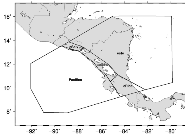
Figura 12. División de la región en zonas de ocurrencia de terremotos superficiales [0, 40) km. Fuente: elaboración propia en base a gnuplot ® (Williams y Kelley, 2017) y el GMT (Wessel y Smith, 1998).
