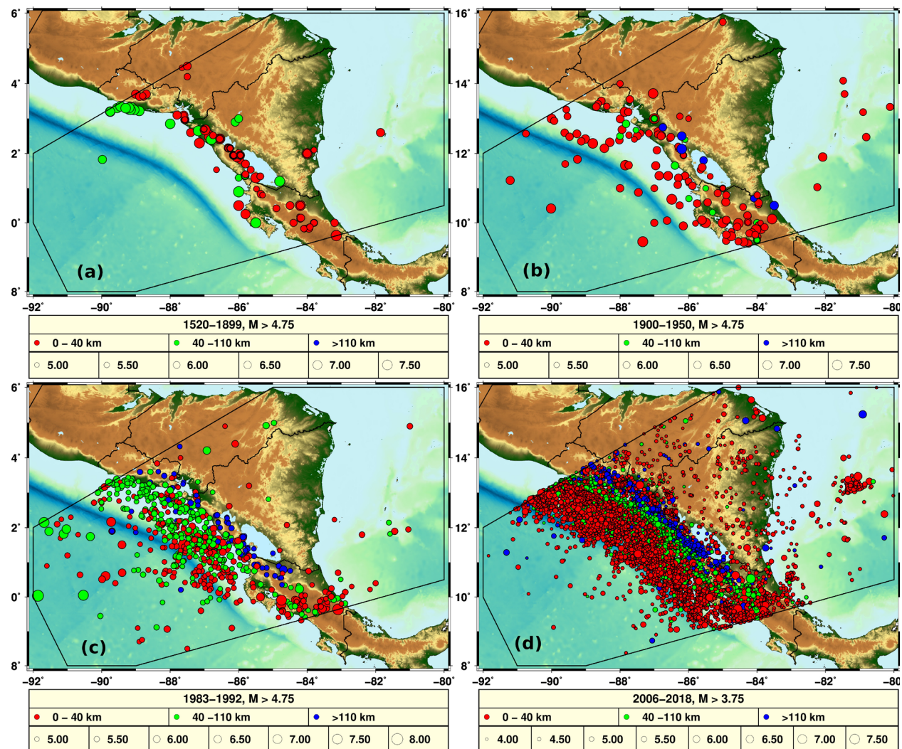
Figura 3. Mapas de epicentros. Fuente: elaboración propia en base a gnuplot ® (Williams y Kelley, 2017) y el GMT (Wessel y Smith, 1998).
