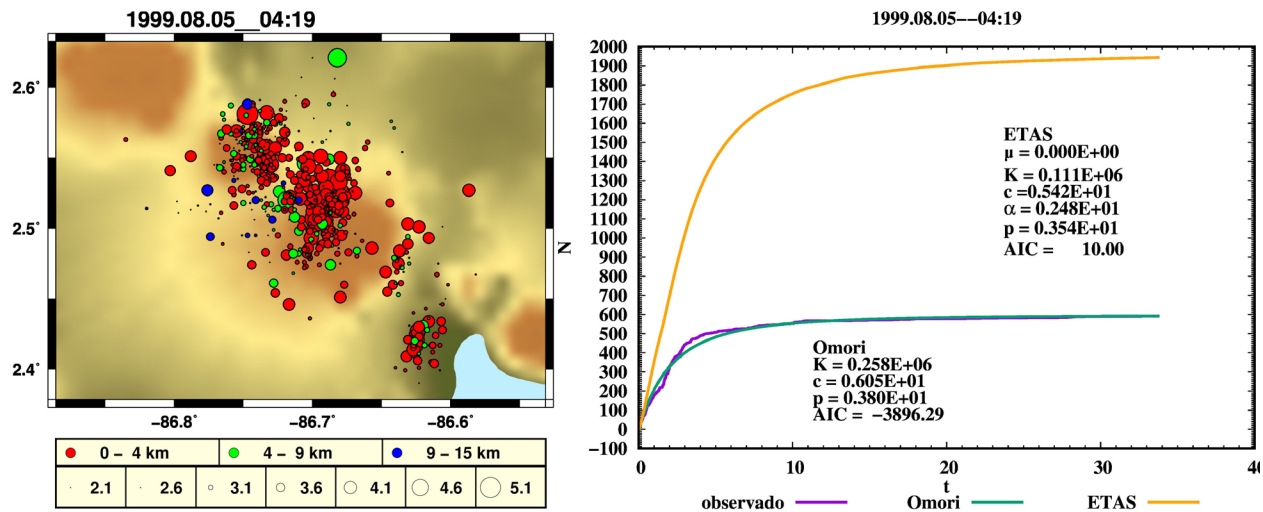
Figura 4. Agrupamiento de terremotos en los alrededores del volcán Cerro negro (1999). Fuente: elaboración propia en base a gnuplot ® (Williams y Kelley, 2017) y el GMT (Wessel y Smith, 1998).
