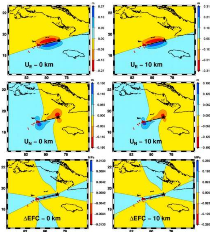
Figura 9. Resultados de la aplicación del programa PSGRN/PSCMP (Wang et al., 2006). Aparecen: 1) estrella negra (epicentro del terremoto principal); 2) línea negra (la falla); 3) puntos rojos (epicentros de las réplicas); 4) UE=Deslizamiento E-O, UN=Deslizamiento N-S, \Delta EFC =Esfuerzo de fractura de Coulomb.
